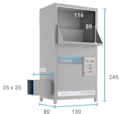
CARDBOXPRESS 200 MIT LADEÖFFNUNG
