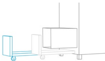
Schublade mit STOPP-Funktion
