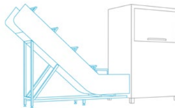
Direkter Ladeausgangskanal in den 1100-L-Behälter
