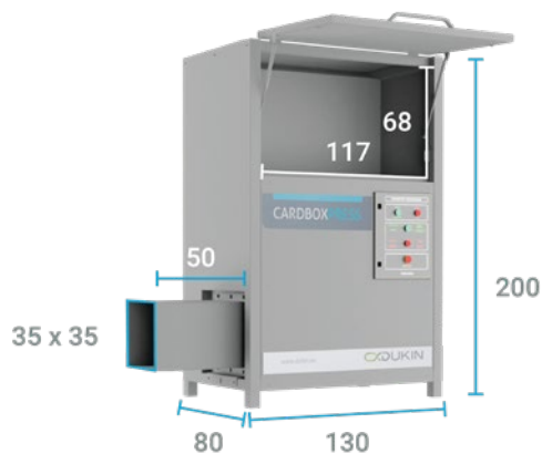
CARDBOXPRESS 200 MIT DECKEL
