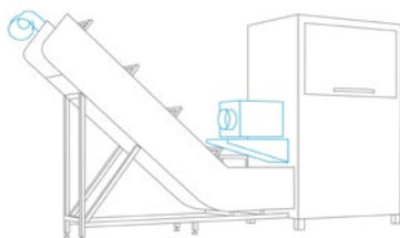
Direkter Ladeausgangskanal in den 1100-L-Behälter mit Staubpartikelfiltrationssystem
